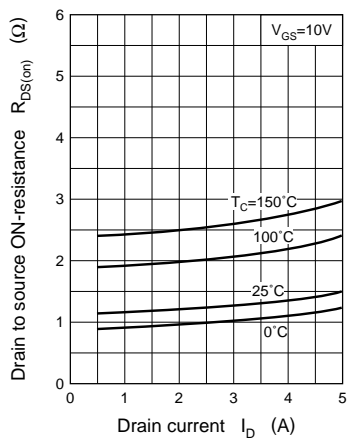
R_{DS(on)} - I_D
