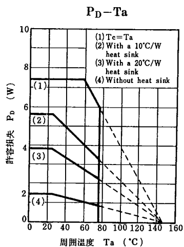
AN6535 特性図
